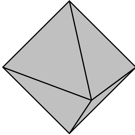
Un octaedro
