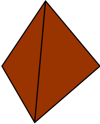
Un tetraedro
