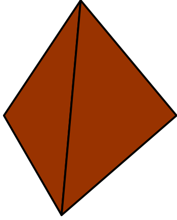
Bir dört yüzlü
