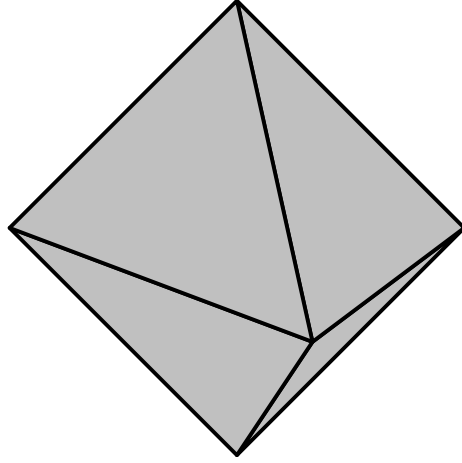
Bir sekiz yüzlü
