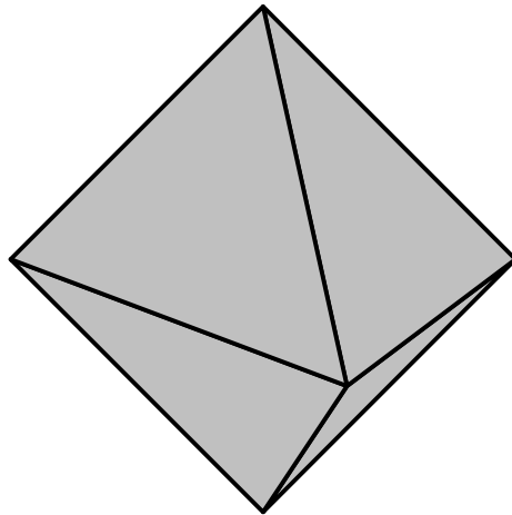
Ein Oktaeder
