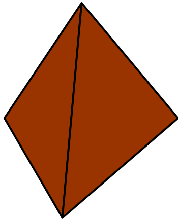
Ein Tetraeder
